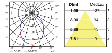
LED Blanco cálido / Warm white
