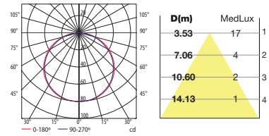
91-0150-00-00 LED Blanco cálido / Warm white
