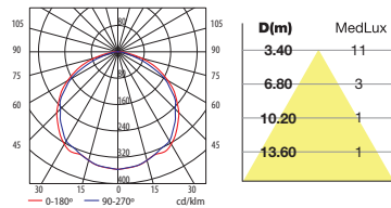
91-3420 LED Blanco cálido / Warm white
