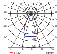
HIT-T G12 70W 45°
