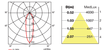
HIT-T G12 70W 45°
