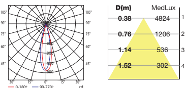
DELTA 6 LED Blanco cálido / Warm white 700 mA
