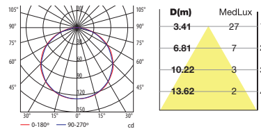
91-4671 LED Blanco cálido / Warm white
