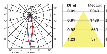
CDM-TM PGJ5 35W 12°
