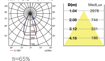
HIT-T G12 70W 45°
