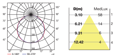
15-4725 LED Blanco cálido / Warm white 1050mA
