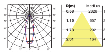
CDM-TM PGJ5 35W 24°
