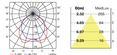
TC-DEL G24q-3 2x26W
