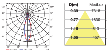
DELTA 9 LED Blanco cálido / Warm white 700 mA
