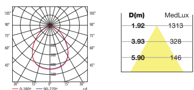
Max. 39W Blanco cálido / Warm white 1900mA
