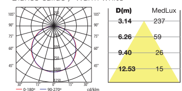
15-2921-52-M1 LED Blanco cálido / Warm white
