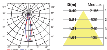
DELTA 3 LED Blanco cálido / Warm white 700 mA
