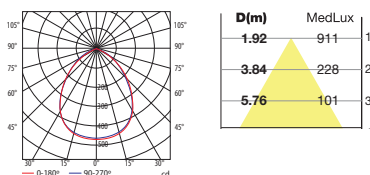
Max. 27W Blanco cálido / Warm white 2000mA
