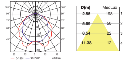
TC-D G24d-3 2x26W
