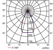
HIT-T G12 70W 45°
