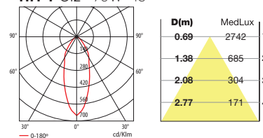
HIT-T G12 70W 45°
