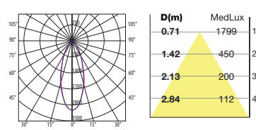
CDM-TM PGJ5 35W 38°
