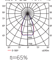
HIT-T G12 70W 45°
