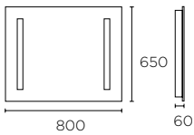
426-ES 2 X 2G11 55W
