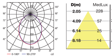
LED Blanco cálido / Warm white
