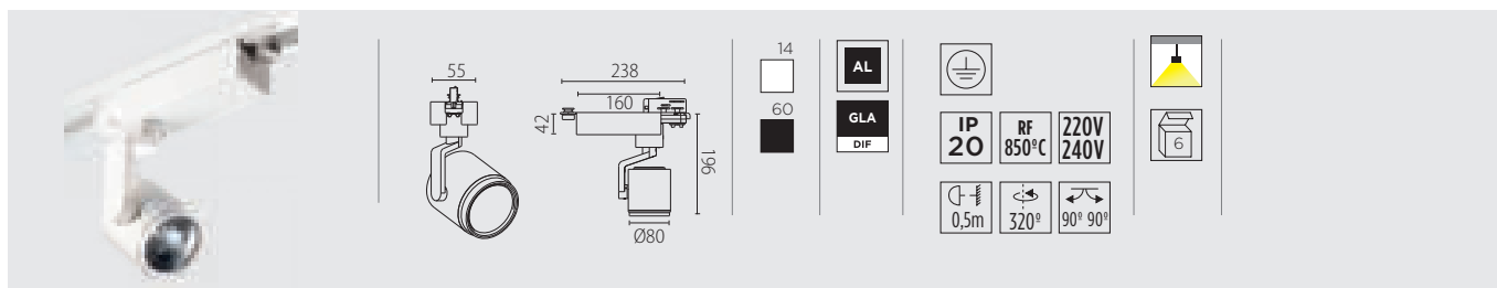
CDM-TM PGJ5 35W 12°
