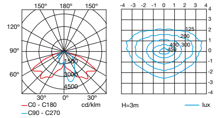
HPS 70W ULOR INST = 0,1%
